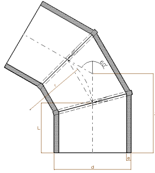
KONFEKSİYON 60 ° DİRSEK SEGMENTED 60 ° ELBOW PE100 - SDR 17 - PN10 ve SDR 11 - PN16
